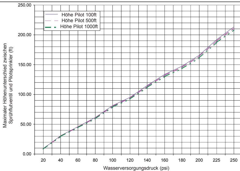
Abbildung 64 - DN200 (8'') SPRÜHFLUTVENTIL MODEL F-1
