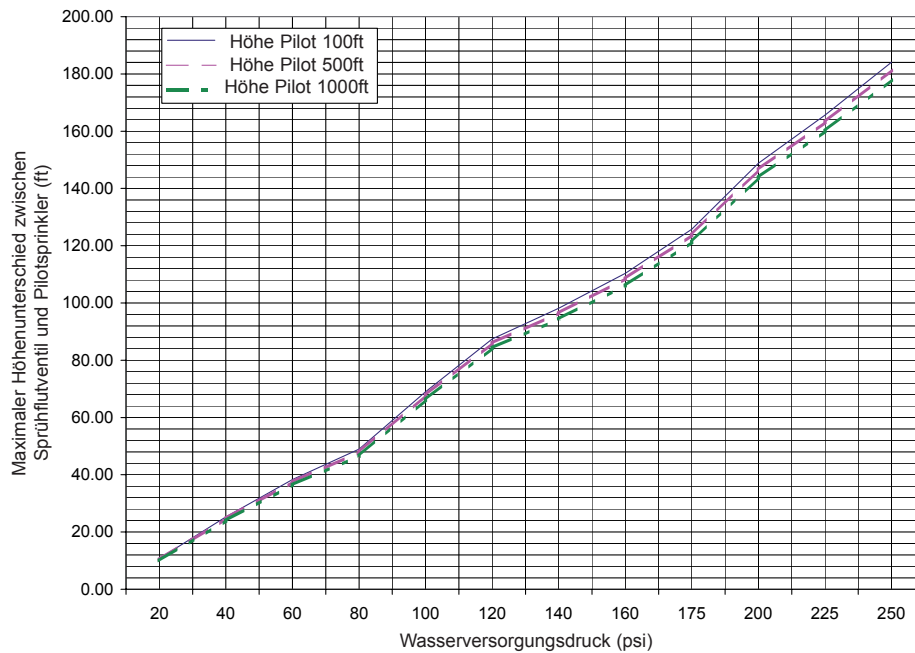
Abbildung 5 - DN150 (6'') SPRÜHFLUTVENTIL MODEL F-1
