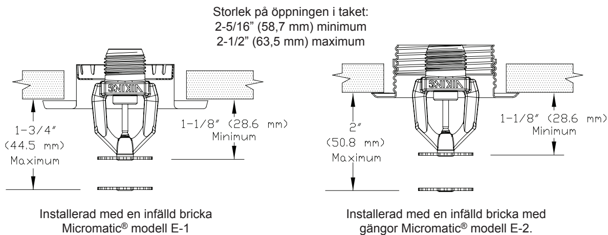
Bild 4: Sprinkler VK4660 dimensioner med modell E-1 och E-2 infällda brickor
