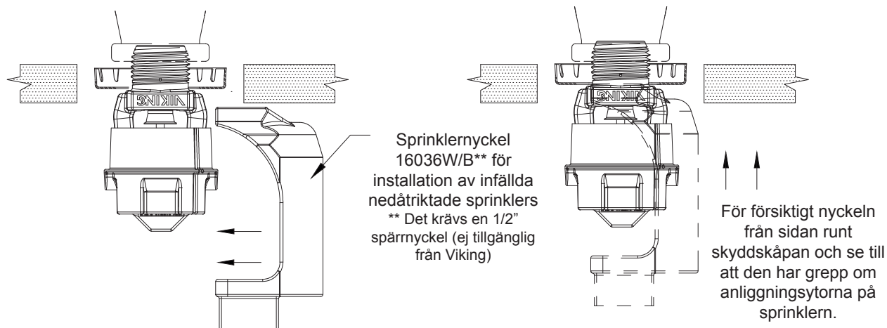
Bild 2: Nyckel 16036W/B för belagd och/eller infälld sprinkler VK4660
