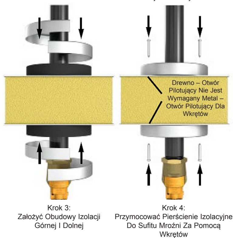
Rysunek nr 1: Montaż pierścieni izolacyjnych tryskacza wiszącego suchego ESFR z przyłączem rowkowanym
