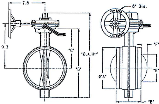
01G 8" SHOWN
